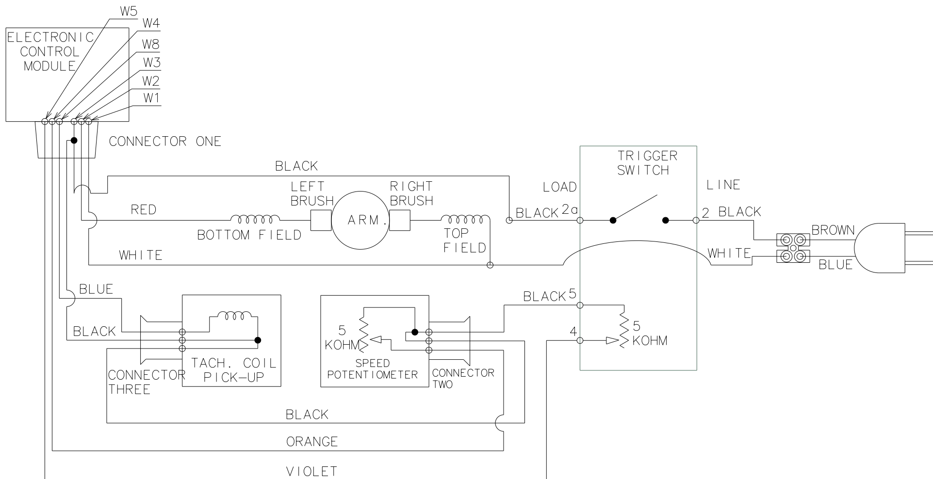
WIRING SCHEMATIC
